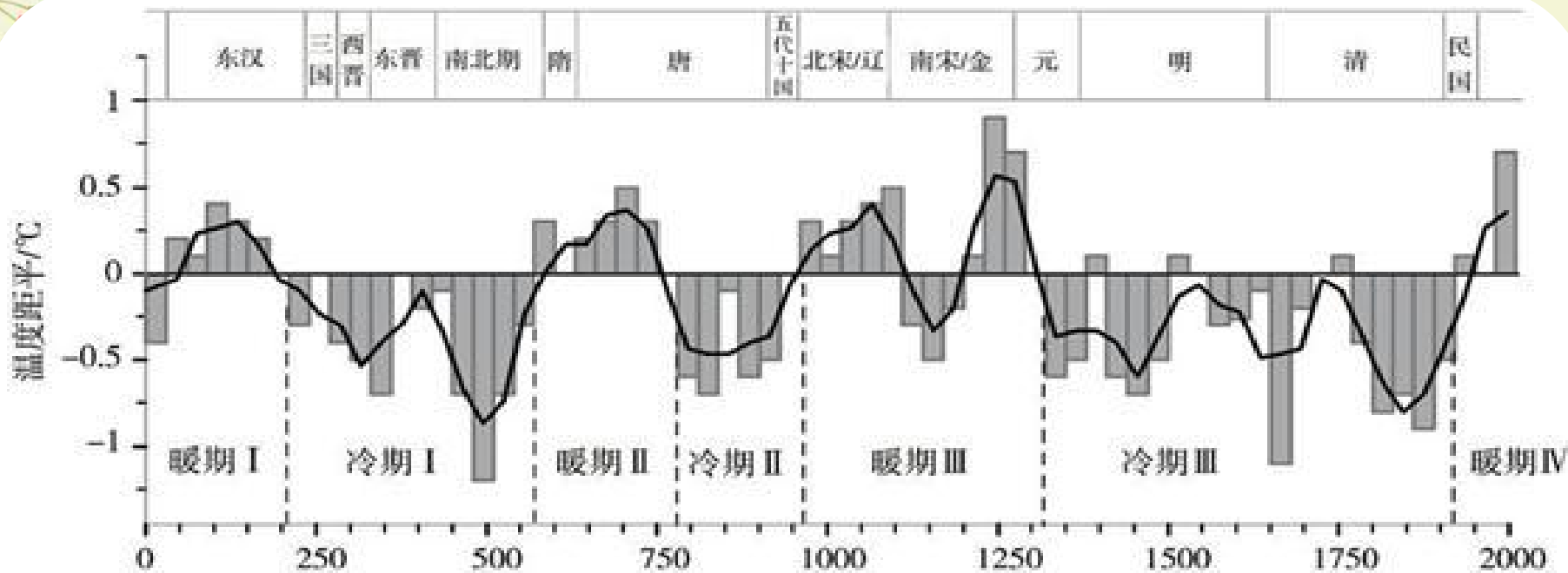
图1 历史时期中国东部冬半年平均温度变化曲线 (温度距平数据引自文献 [17])
